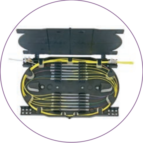
Opsiyon 2 Splice Tepsisinin Kaseti, İç Görünüm
