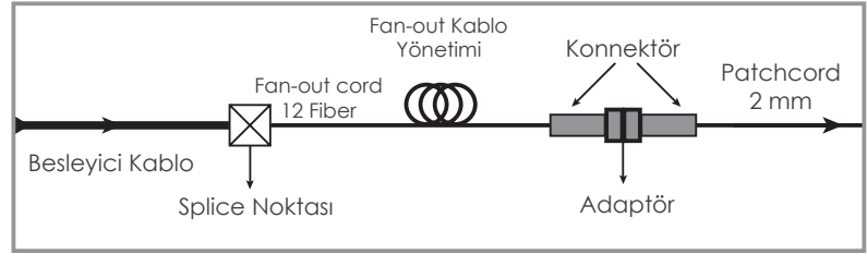
PERGE ODF Modülü İşlevsel Blok Diyagramı
